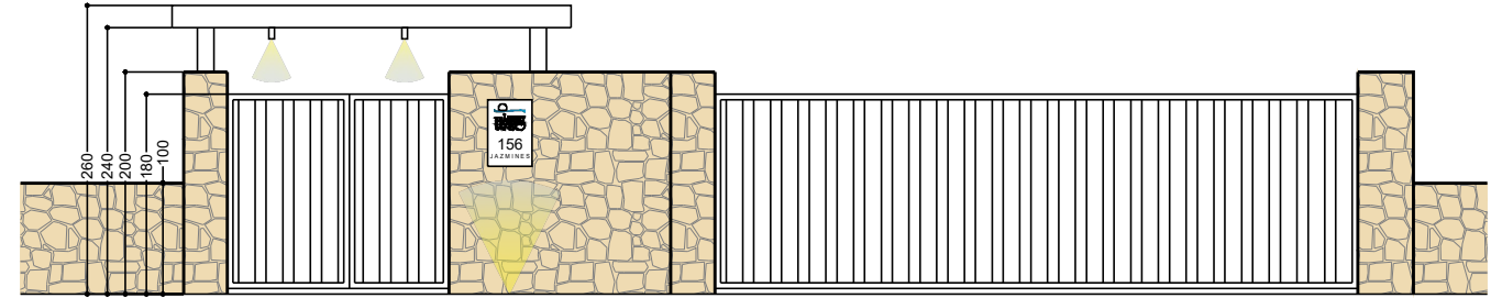
DETALLE ENTRADA
